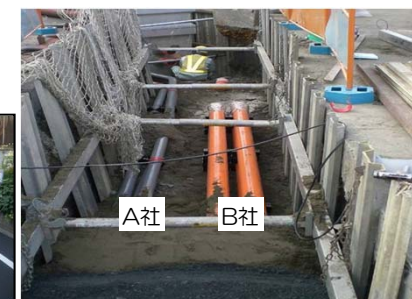
「土工工程の共同施工」
